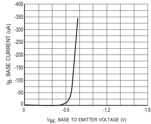
Figure4 I_B - V_{BE}
