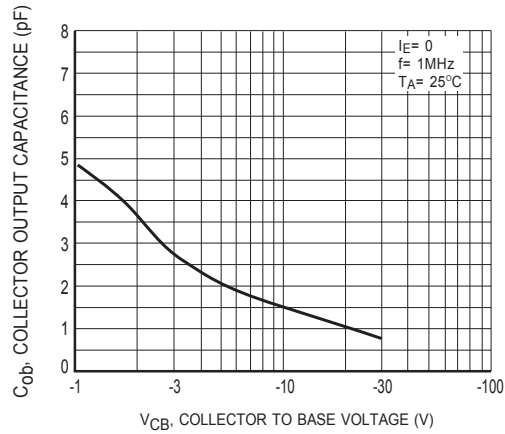
Figure9 C_{ob}-V_{CB}
