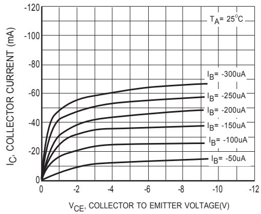
Figure2 I_C - V_{CE}
