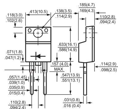
ITO-220A
